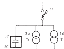
▶ 一括保護設備の単結線図
