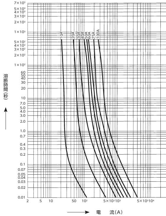
PF形 (7.2kV) 溶断時間—電流特性
