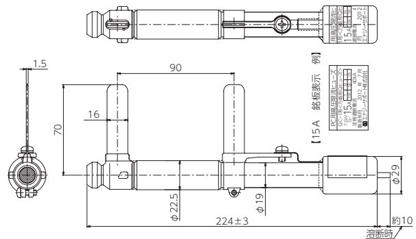
外形図
