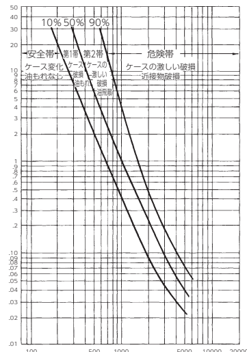
200Kvar コンデンサ破壊確率曲線
