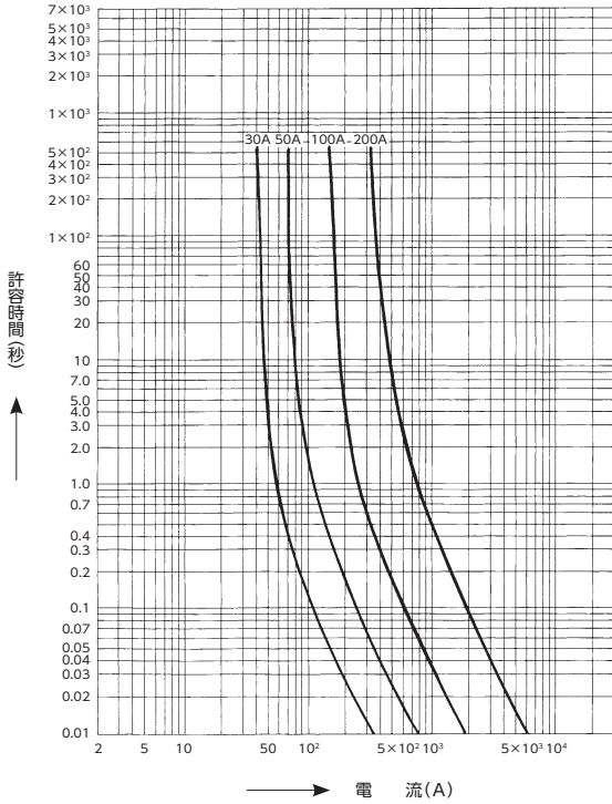
PFG-1C 形 (3.6kV) 許容時間—電流特性
