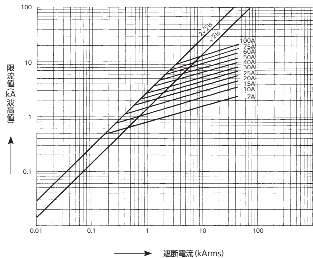
PFU-1 形 (7.2kV) 限流特性
