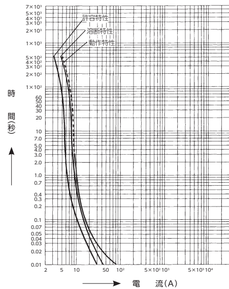
QPT-1 形の時間—電流特性
