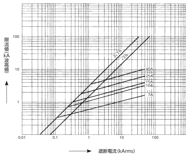
QC-1、QCC-1 形 (7.2kV) 限流特性
