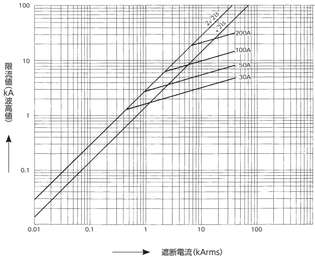
PFG-1C 形 (3.6kV) 限流特性
