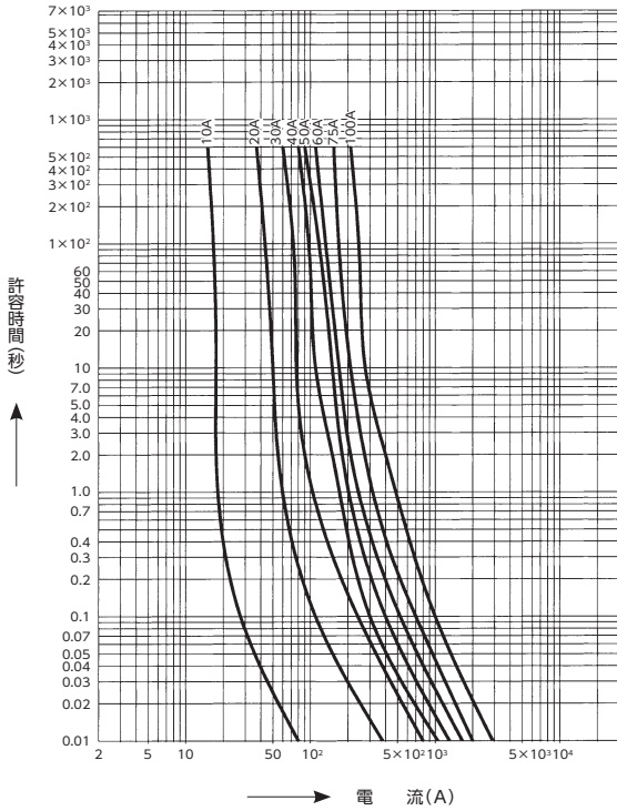
PF形 (7.2kV) 許容時間—電流特性
