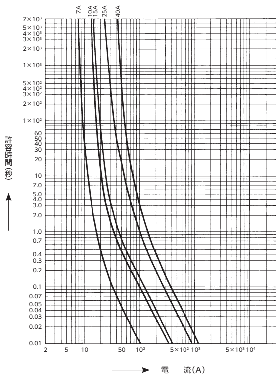
QC-1、QCC-1 形 (7.2kV) 許容時間—電流特性
