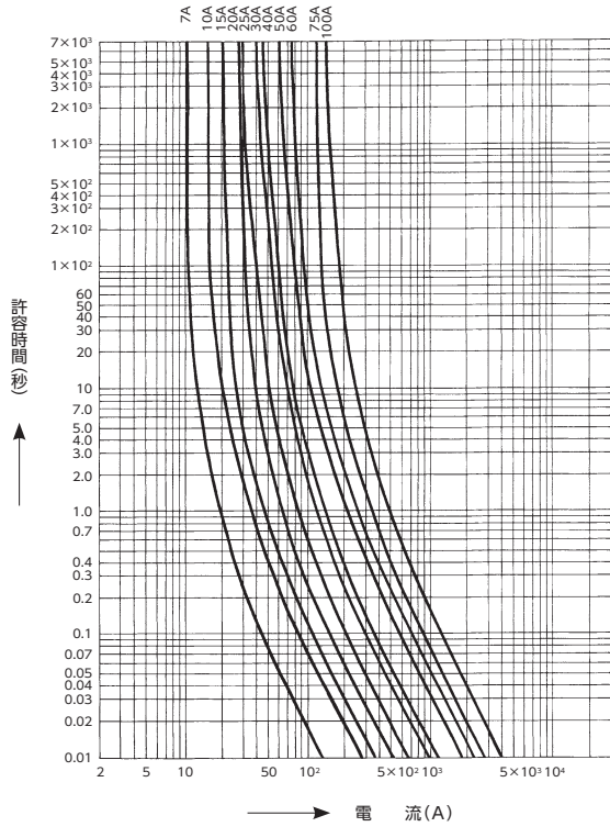
PFU-1 形 (7.2kV) 許容時間—電流特性
