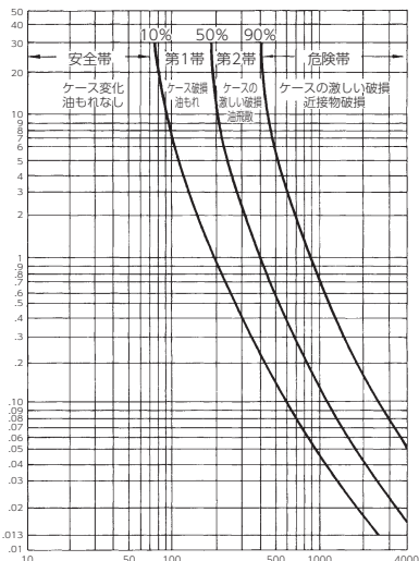
50Kvar コンデンサ破壊確率曲線
