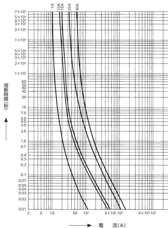
QC-1、QCC-1 形 (7.2kV) 溶断時間—電流特性
