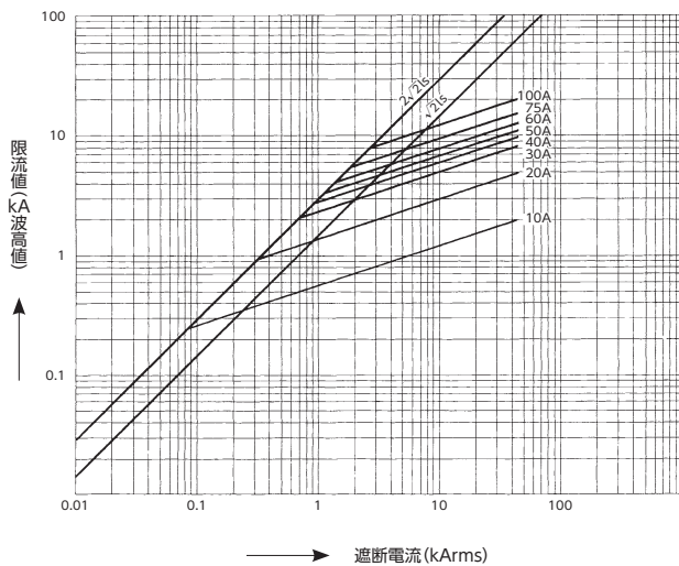
PF形 (7.2kV) 限流特性
