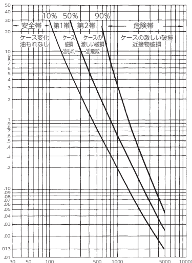
100Kvar コンデンサ破壊確率曲線
