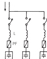
図2 直列リアクトルの設置
