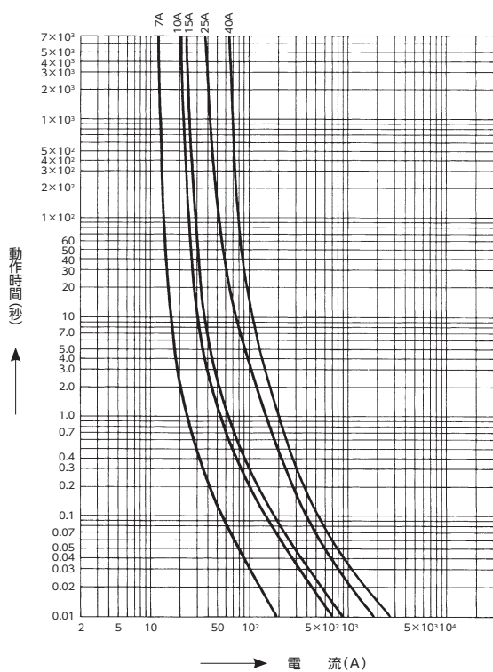
QC-1、QCC-1 形 (7.2kV) 動作時間—電流特性
