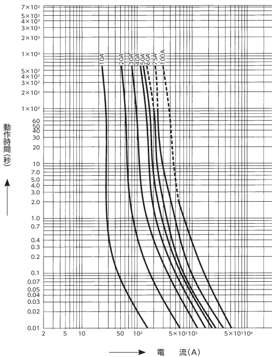
PF形 (7.2kV) 動作時間—電流特性
