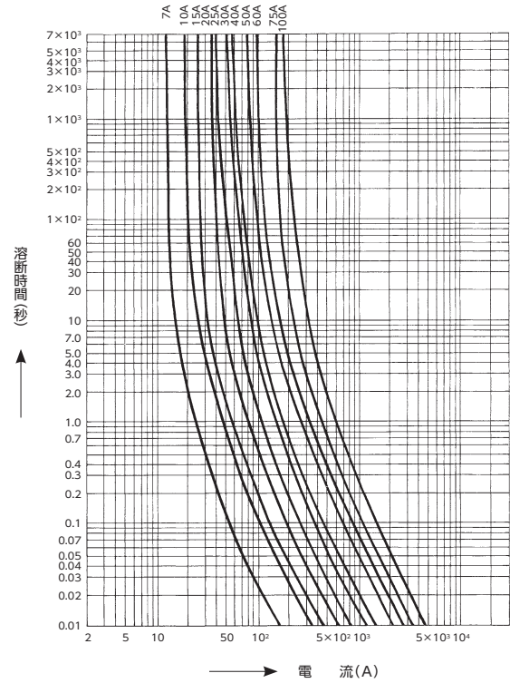
PFU-1 形 (7.2kV) 溶断時間—電流特性
