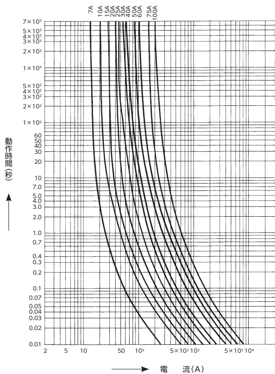
PFU-1 形 (7.2kV) 動作時間—電流特性
