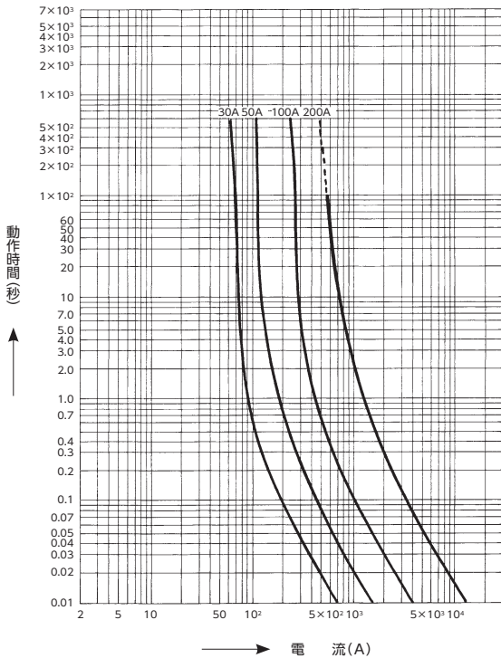
PFG-1C 形 (3.6kV) 動作時間—電流特性
