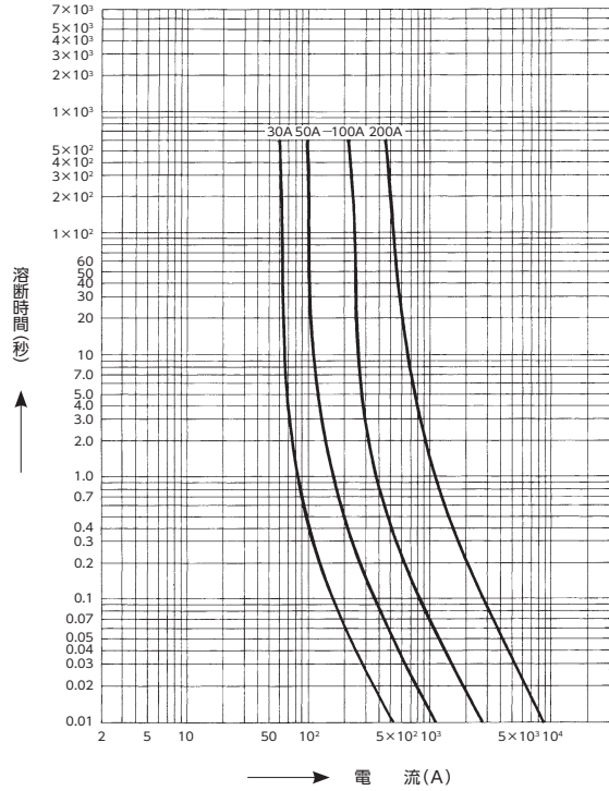
PFG-1C 形 (3.6kV) 溶断時間—電流特性
