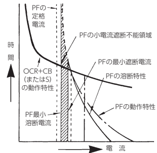
▶ 電力ヒューズと過電流継続器の協調
