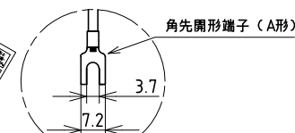
B 詳細図 (拡大)
